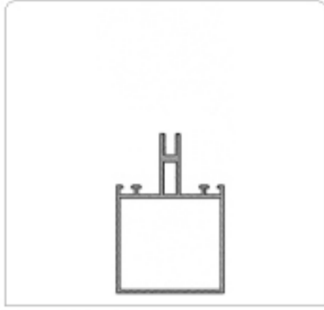
FMG-1611 50'LİK CEPHE 1.6 MM
