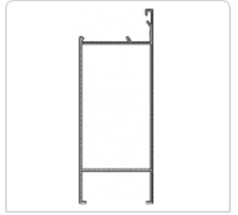
FMG-2014 ETEK PROFİLİ
