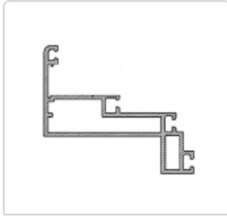
FMG-1621 SAKLI KANAT KASA PROFİLİ
