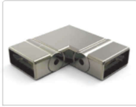
FMG-137 80X30 DİRSEK ÇİFT TARAF OYNARLI 90°
