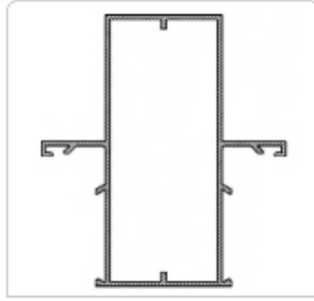
FMG-2009 KILIÇ KASA
