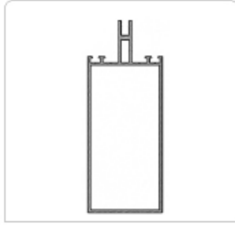
FMG-1613 105'LİK CEPHE 1.8 MM
